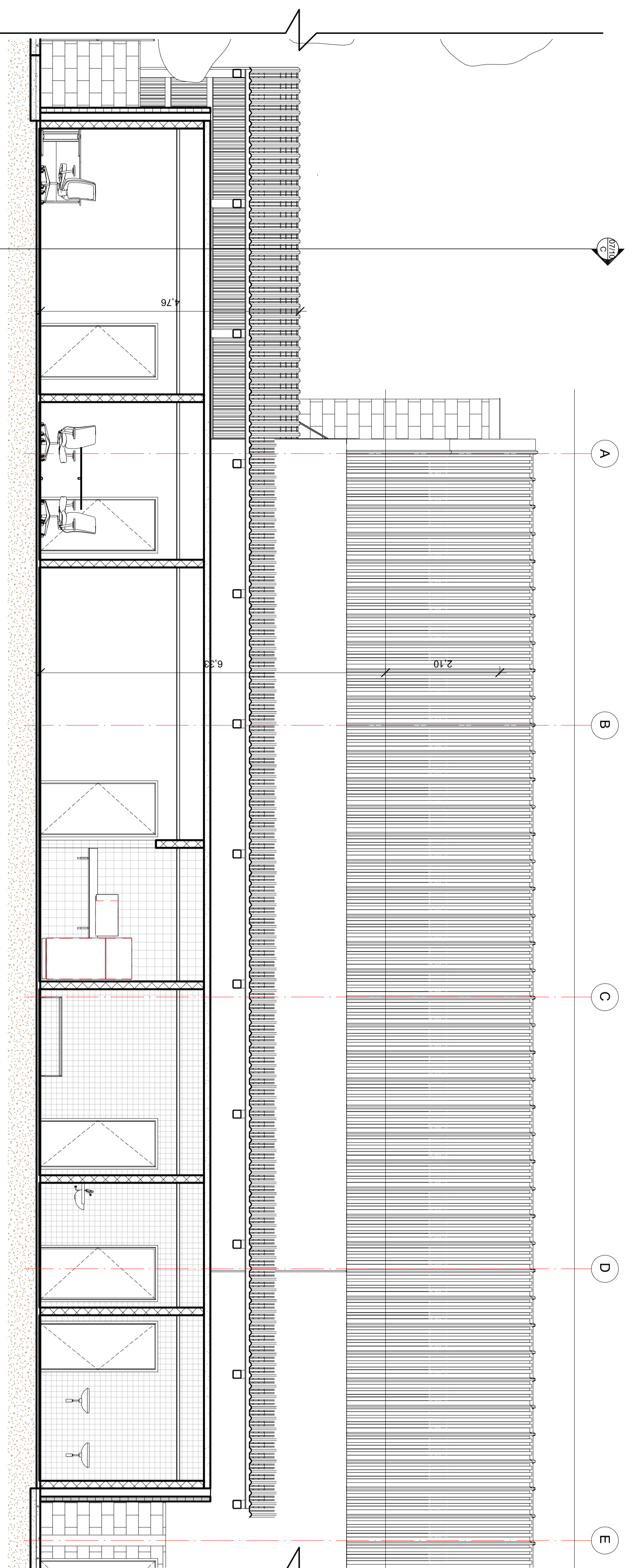
D COMPLETA 1:30
